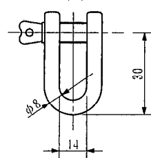
[※] SHACKLE シャックル
