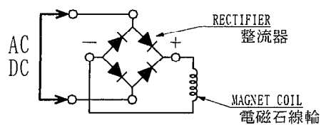
CONNECTION DIAGRAM 結線図
